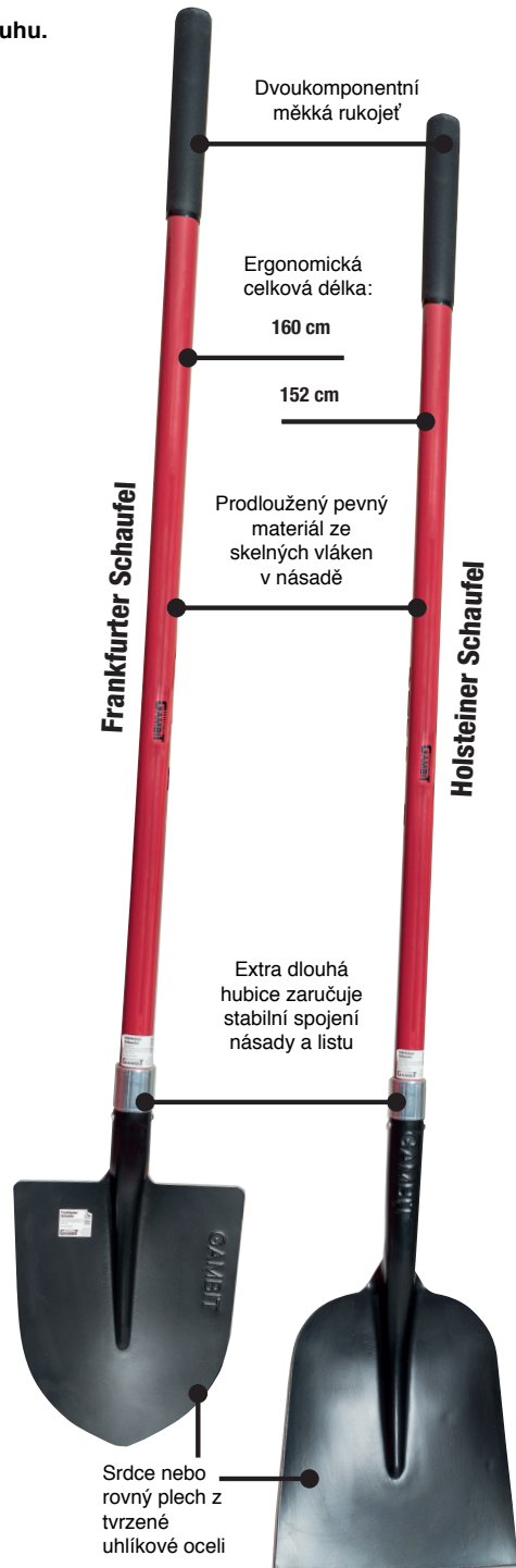
Frankfurtská a Holštýnská lopata: Robustní čepel a pružná rukojeť vydrží i extrémní zatížení v páce.
